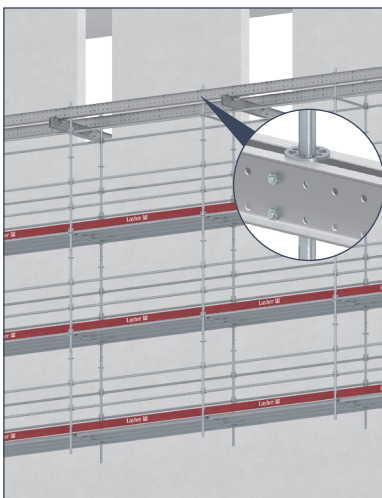
Andamio suspendido de Viga Twix.
