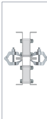
Vigas colocadas una sobre otra aseguradas con grapas para viga (izquierda) o con separador (derecha).
