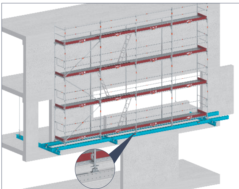
Andamio en voladizo, sobre estructura de Viga Twix montada en forma de rejilla y arriestrada contra la losa.
