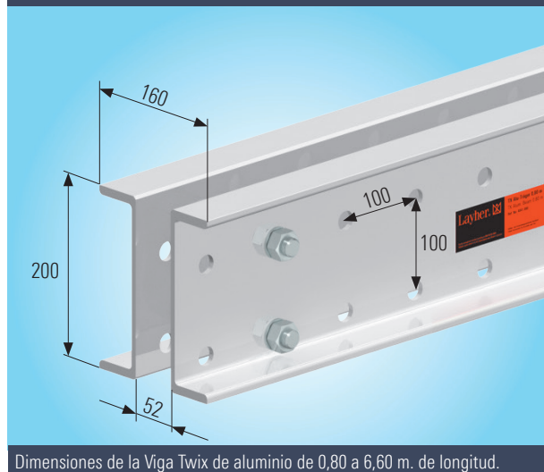
Sección transversal de la Viga Twix de aluminio.
