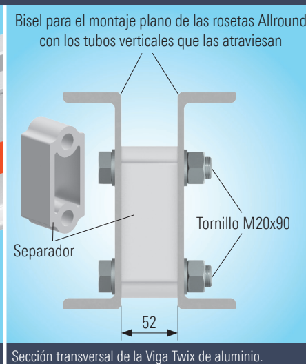
Uso con vertical Allround pasante.
