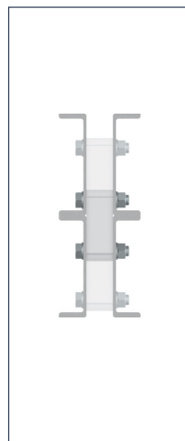
Vigas colocadas una sobre otra aseguradas con grapas para viga (izquierda) o con separador (derecha).
