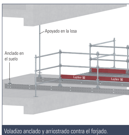
Voladizo anclado y arriestrado contra el forjado.
