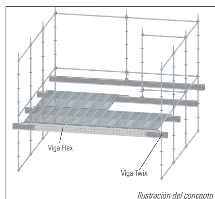
Estructura híbrida de Viga Twix y Viga Flex.
